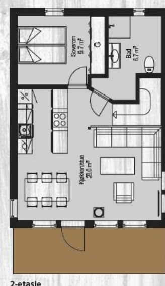
2-etasje
